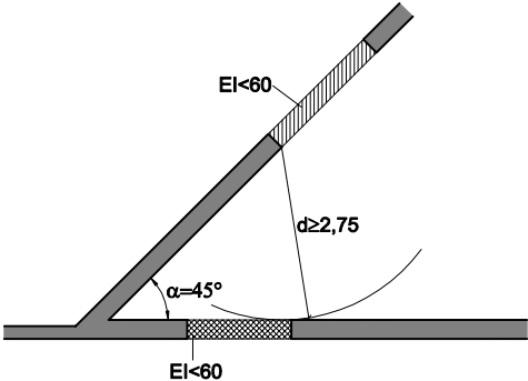
Figura 1.2. Fachadas a 45 
