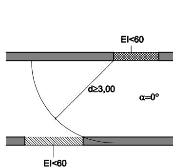
Figura 1.1. Fachadas enfrentadas
